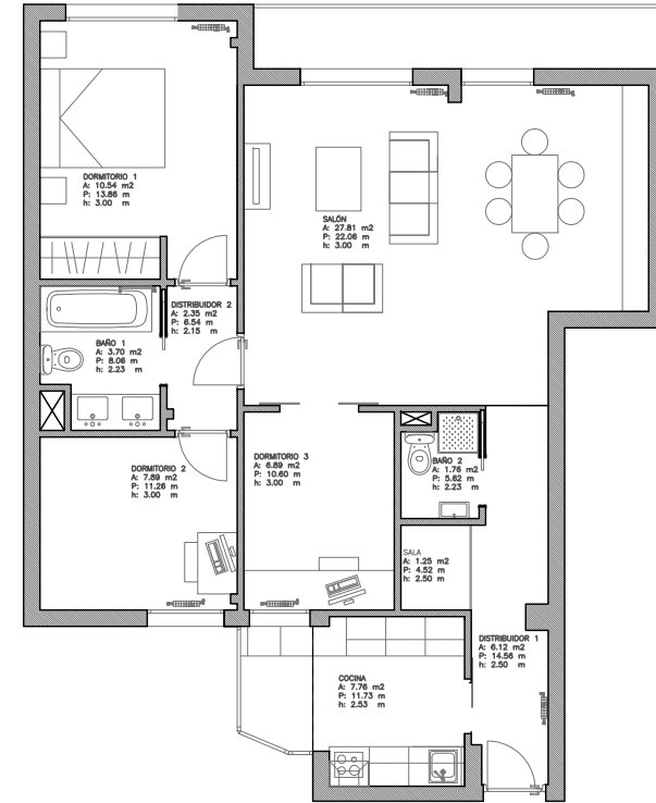
ESTADO REFORMADO
