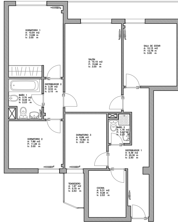
ESTADO PREVIO
